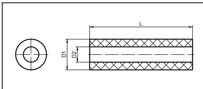
Zeichnung zu PU80., PU90., PU95. Polyurethan-Hohlstäbe
