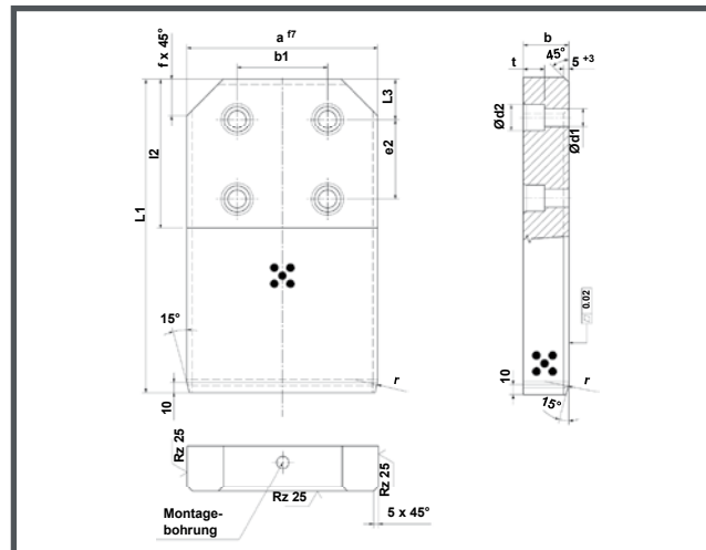
Zeichnung zu 5152. (4 Schrauben ab 140 x 315 mm)
